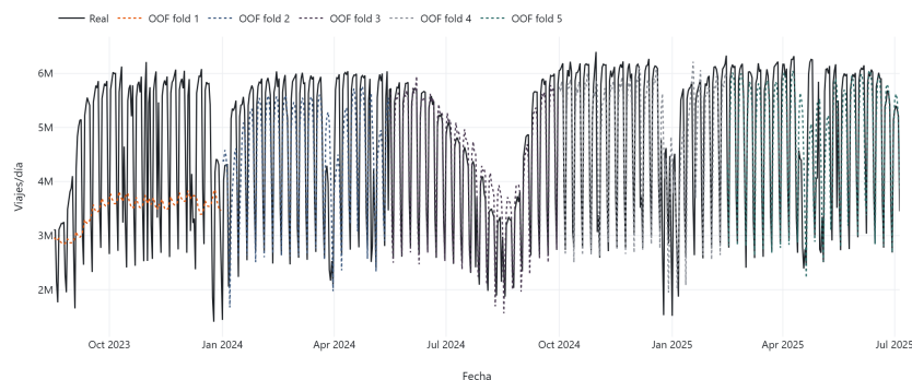
Figura 4.1: Predicción LSTM fuera del pliegue de entrenamiento (OOF) por fold del walk-forward expansivo.
