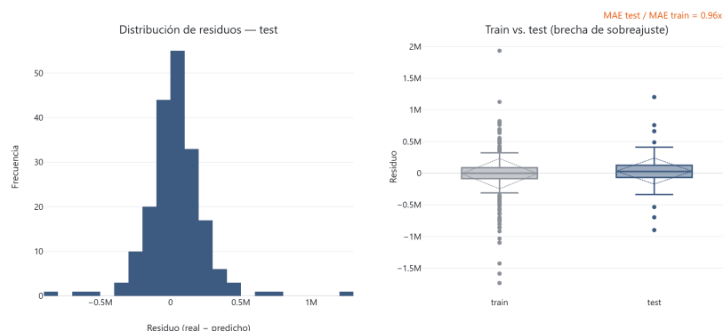
Figura 5.5: Distribución del error de predicción del modelo ensemble_equal (modelo de referencia) en la partición test.
