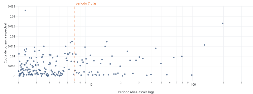
Figura 5.11: Periodograma del residuo de la etapa 1: cuota de potencia espectral frente al periodo en días (escala logarítmica). El periodo de 7 días está anotado; la potencia semanal se dispersa entre bins adyacentes y el armónico de 7/3 días.
