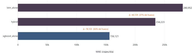
Figura 5.14: Barras escalonadas del MAE de test de los tres modelos de la cadena, con el paso entre barras consecutivas anotado en MAE absoluto y como cuota del hueco total. Deliberadamente no es una cascada con conectores.
