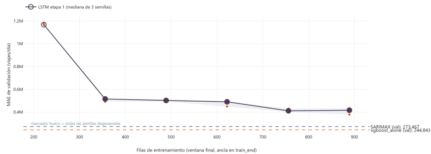
Figura 5.15: MAE de validación de la LSTM de etapa 1 frente a las filas de entrenamiento (ventana descendente anclada en train_end ): mediana y banda mín-máx de 3 semillas (5 en la fracción 1,00), con las líneas de referencia de SARIMAX y xgboost_alone en validación. El marcador hueco indica la fracción cuyas tres semillas degeneraron. La curva se aplana muy por encima de ambas referencias.
