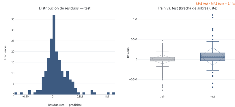
Figura 5.3: Distribución del error de predicción del modelo xgboost_alone en la partición test . La brecha train-test es la evidencia visual del sobreajuste ( R^2 train = 0,9929 frente a MAE test = 156.121).
