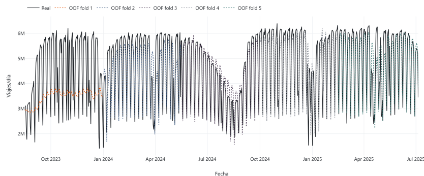
Figura 4.1: Predicción LSTM fuera del pliegue de entrenamiento (OOF) por fold del walk-forward expansivo.
