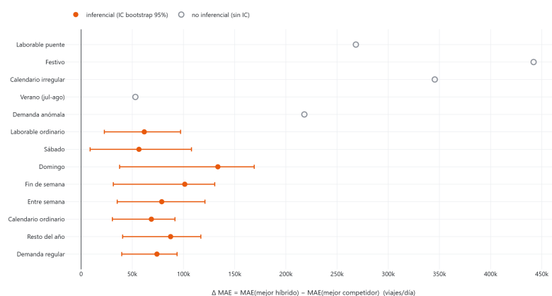
Figura 5.19: Gráfico de bosque de la diferencia de MAE por subgrupo con su IC bootstrap del 95 %. La línea del cero es la referencia: un IC íntegramente a su derecha es evidencia de que el híbrido pierde en ese subgrupo. Marcadores huecos y sin IC para los subgrupos no inferenciales.
