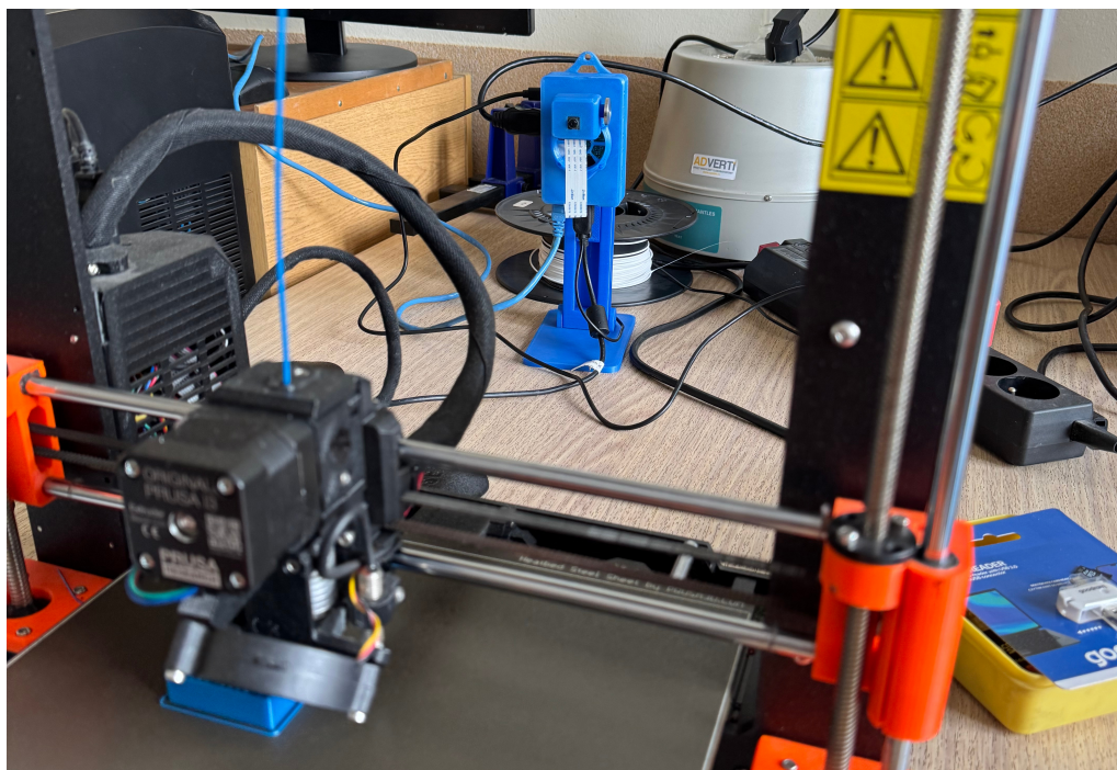
Rysunek 13: Gotowa konstrukcja mechaniczna zainstalowana przy urządzeniu wytwórczym.
