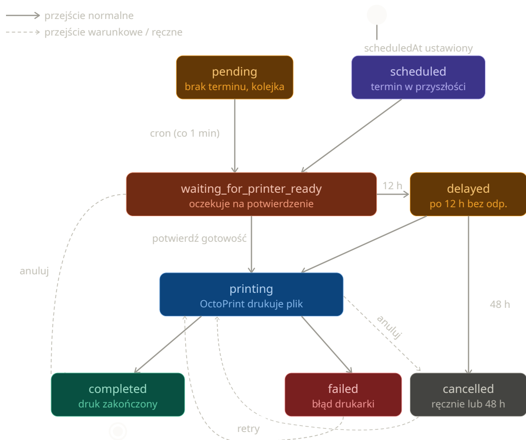
Rysunek 4: Diagram maszyny stanów cyklu życia zadania do wydruku.
