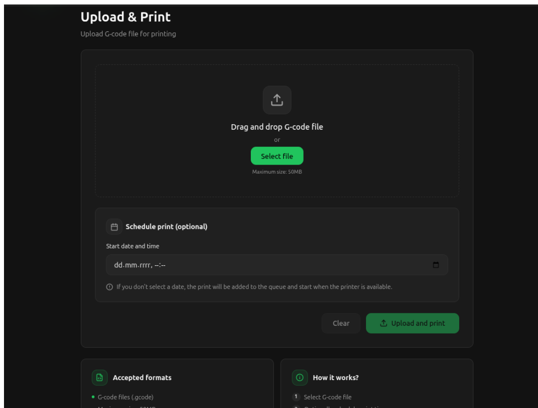
Rysunek 8: Widok panelu przesyłania i planowania zadań w portalu AddiPi .
