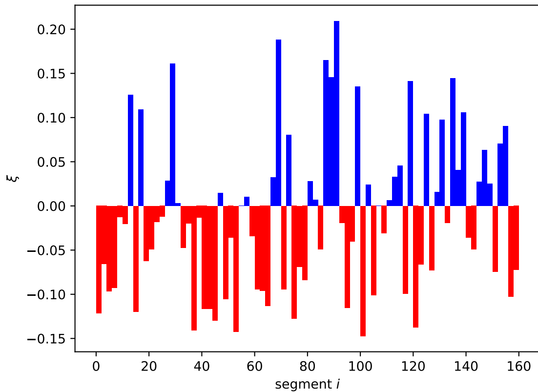
ykgE expression shift \xi_i[11]
