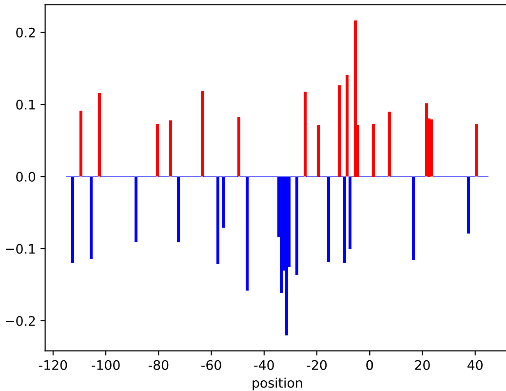
Boostrapped \xi_i
