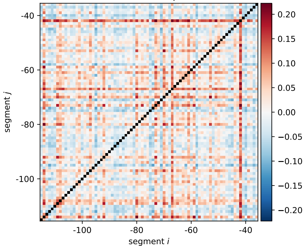
acul expression shift \xi_{i,j}[0011, 1100]
