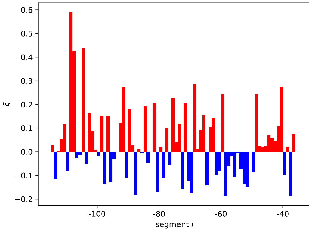
aegA expression shift \xi_i[11]
