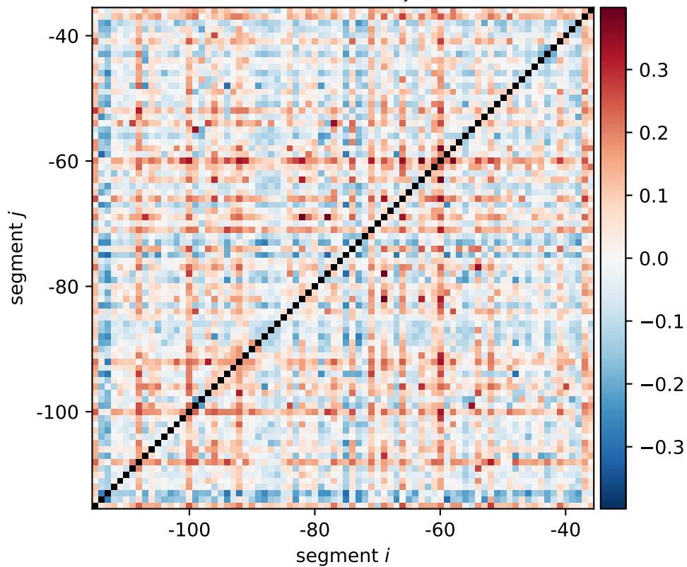
aphA expression shift \xi_{i,j}[0011, 1100]
