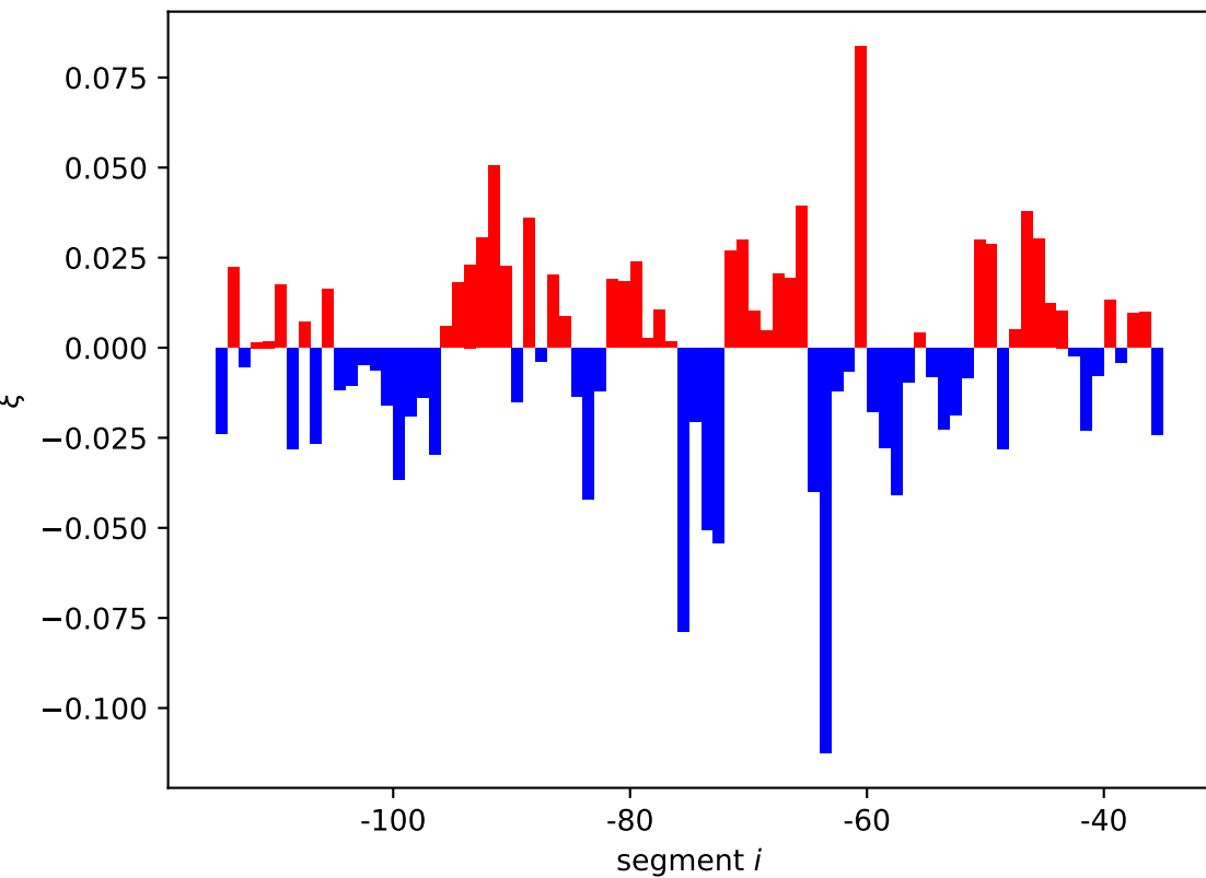
aphA expression shift \xi_i[01, 10]
