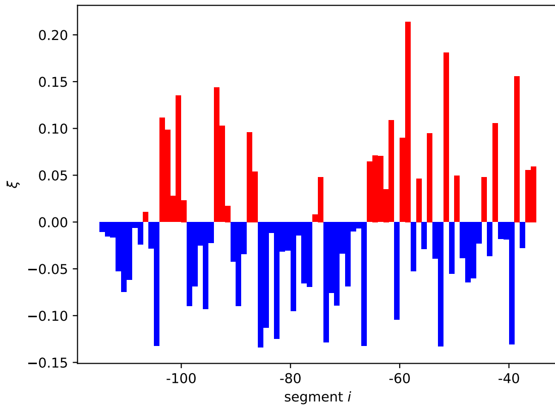
araC expression shift \xi_i[11]
