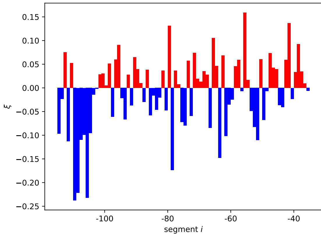
arcA expression shift \xi_i[11]
