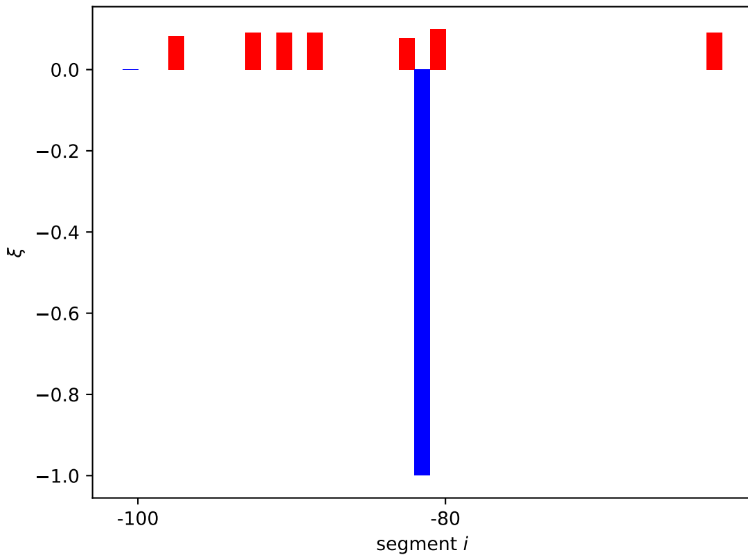
arcB expression shift \xi_i[11]
