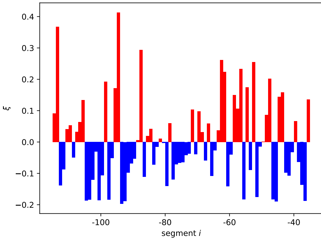
asnA expression shift \xi_i[11]
