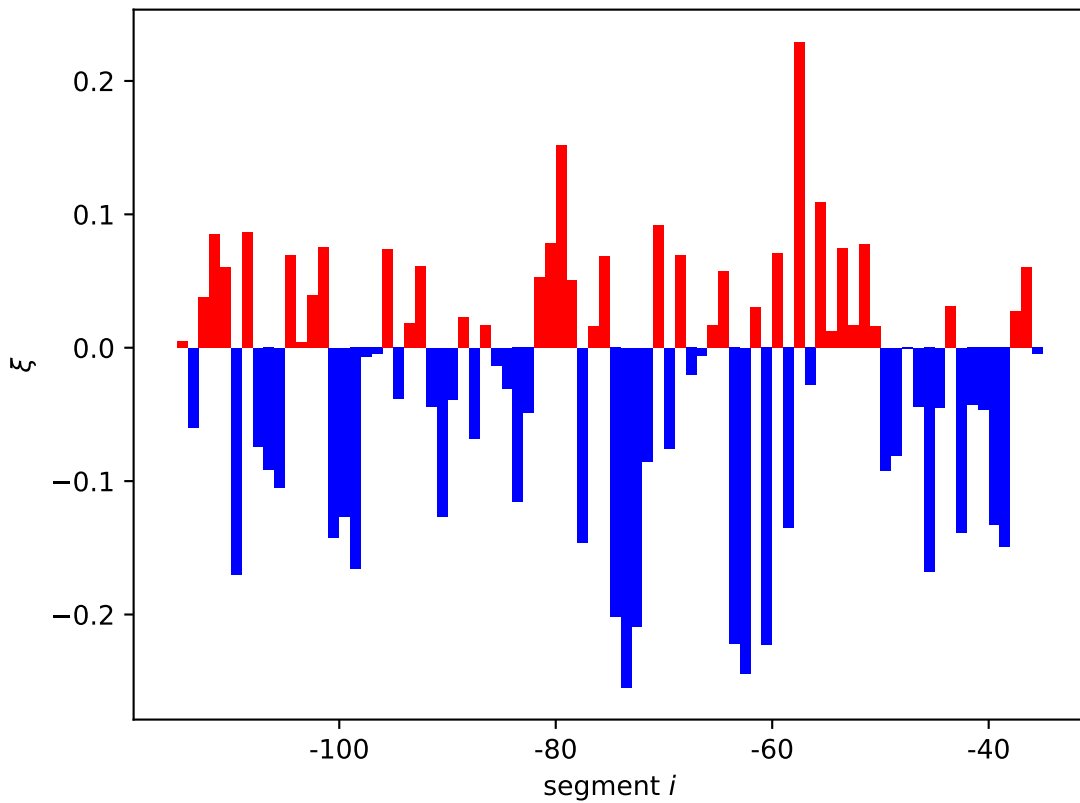
dicC expression shift \xi_i[11]
