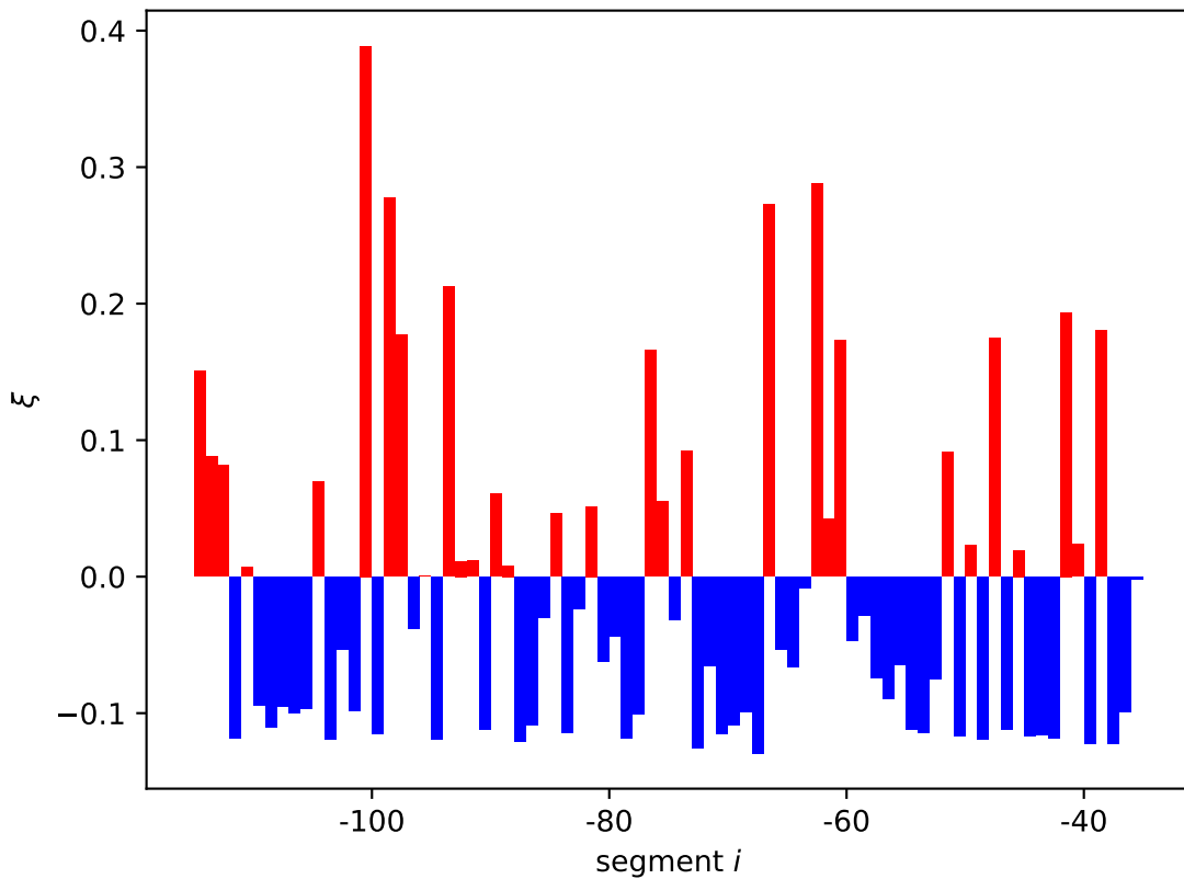
dpiBA expression shift \xi_i[11]
