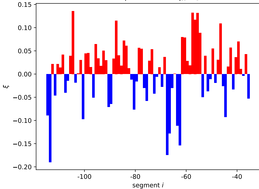
hicB expression shift \xi_i[11]
