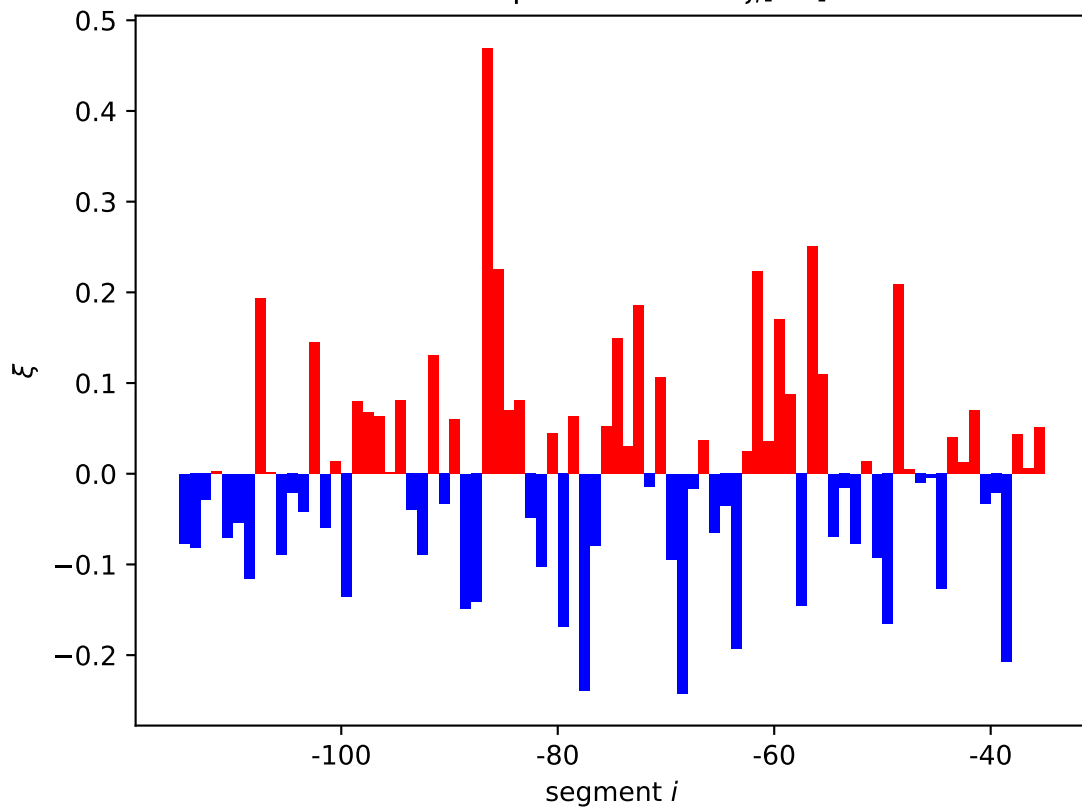
hicB expression shift \xi_i[11]
