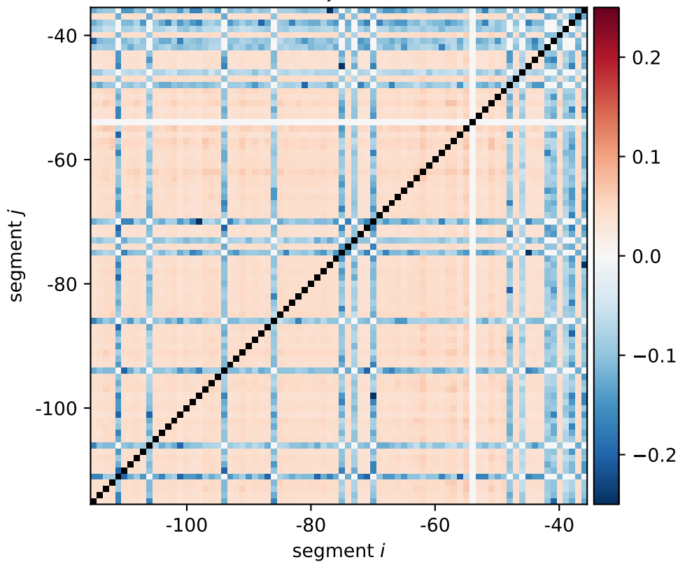
holC expression shift \xi_{i,j}[0001, 0010, 0100, 1000]
