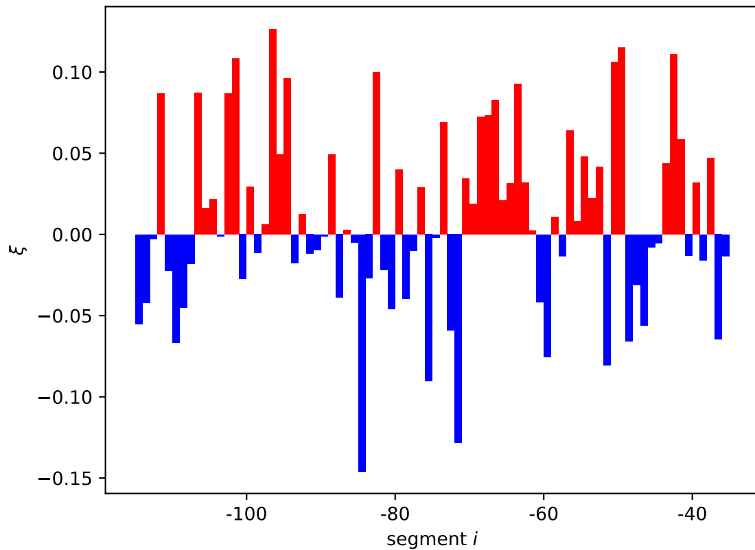
hslU expression shift \xi_i[11]
