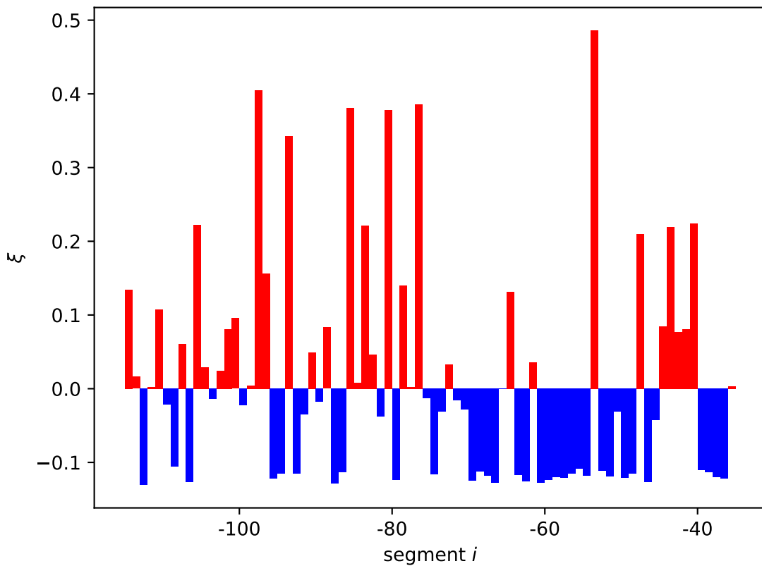
htrB expression shift \xi_i[11]
