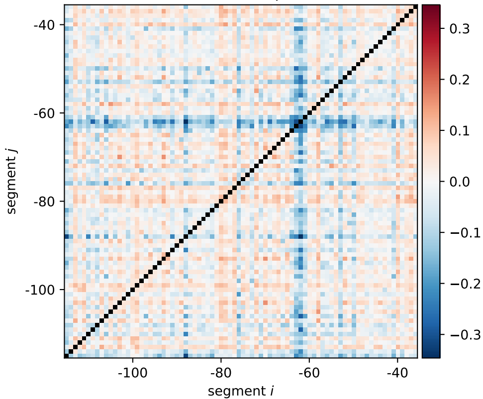
iap expression shift \xi_{i,j}[0011, 1100]
