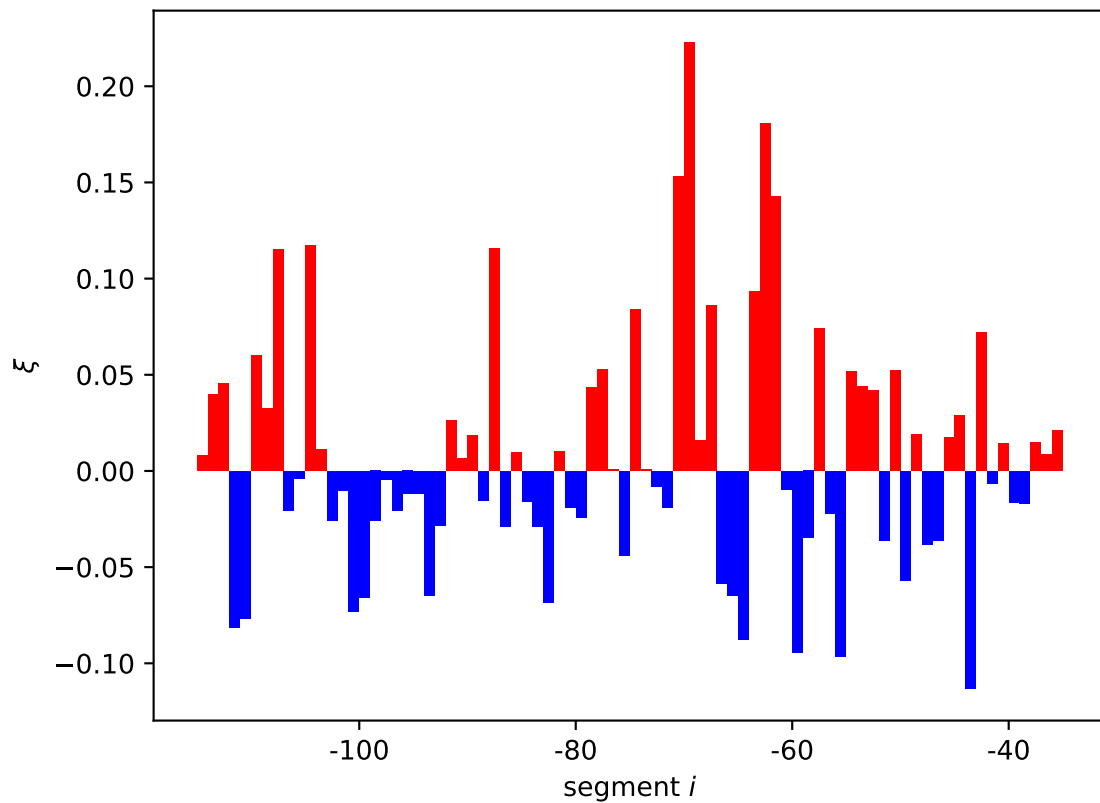
ilvC expression shift \xi_i[11]
