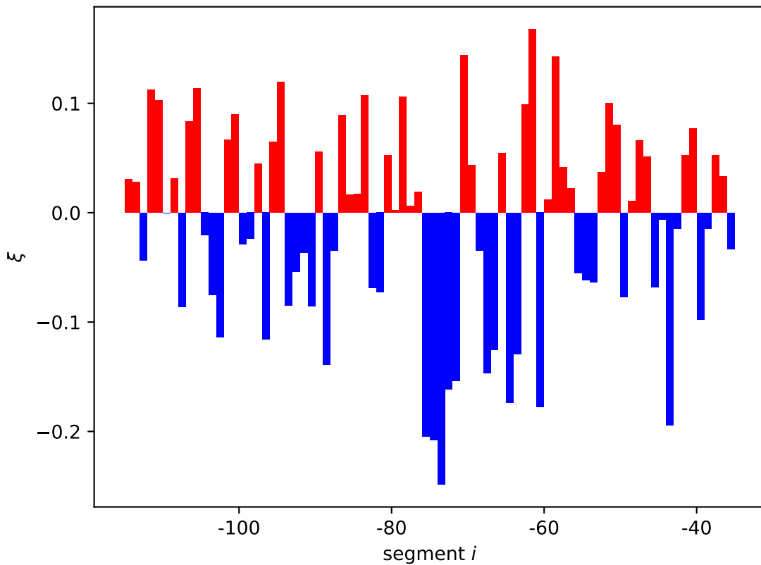
leuABCD expression shift \xi_i[11]
