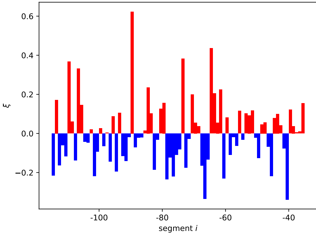
maoP expression shift \xi_i[11]
