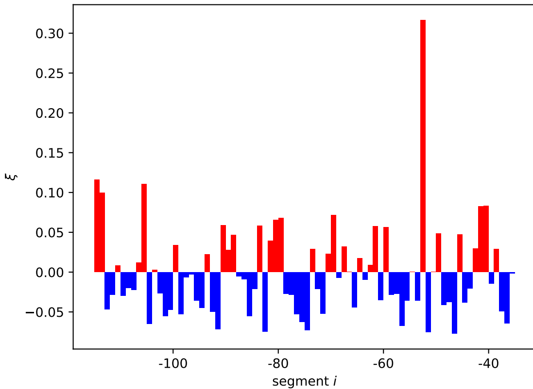
minC expression shift \xi_i[11]
