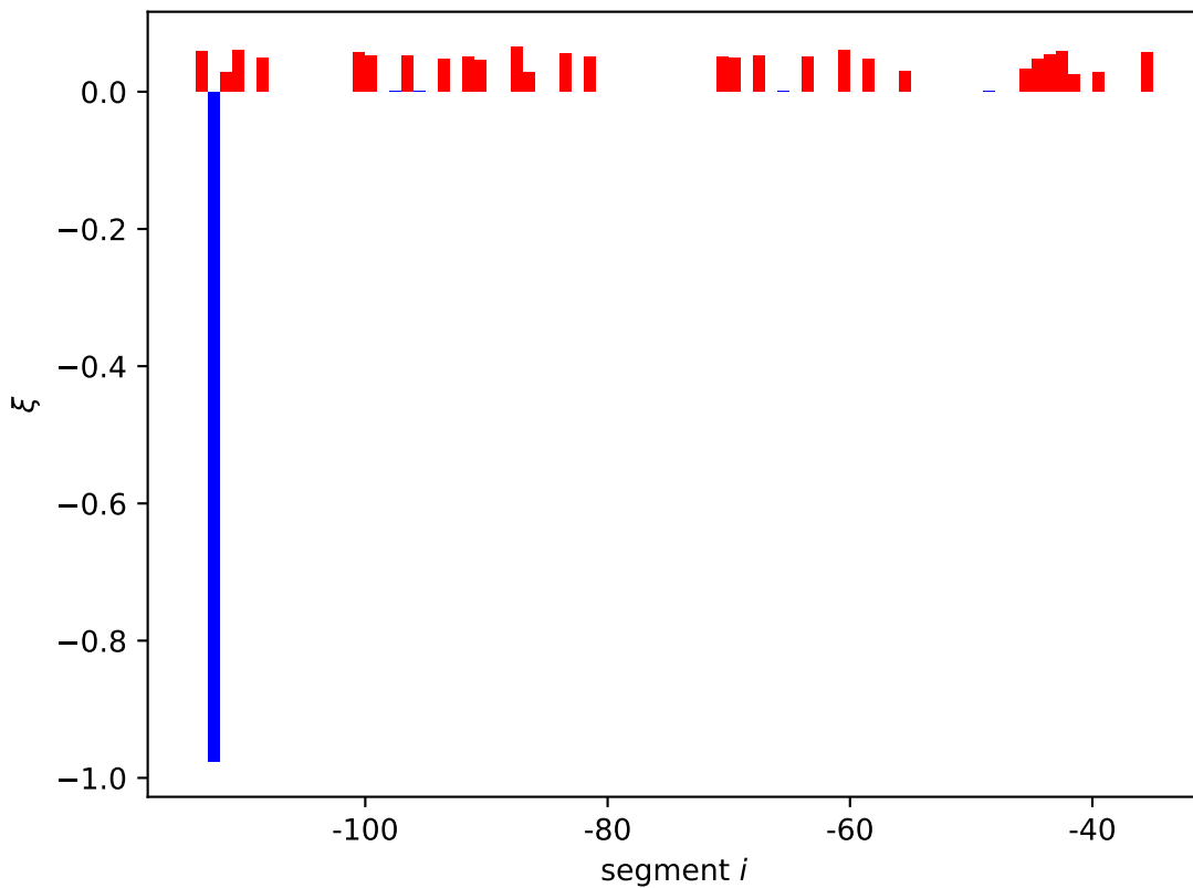
mscK expression shift \xi_i[11]
