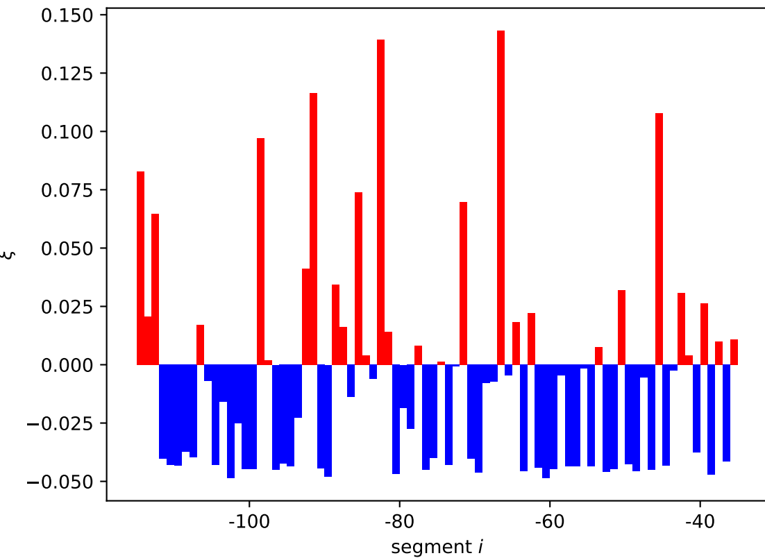
mscL expression shift \xi_i[11]
