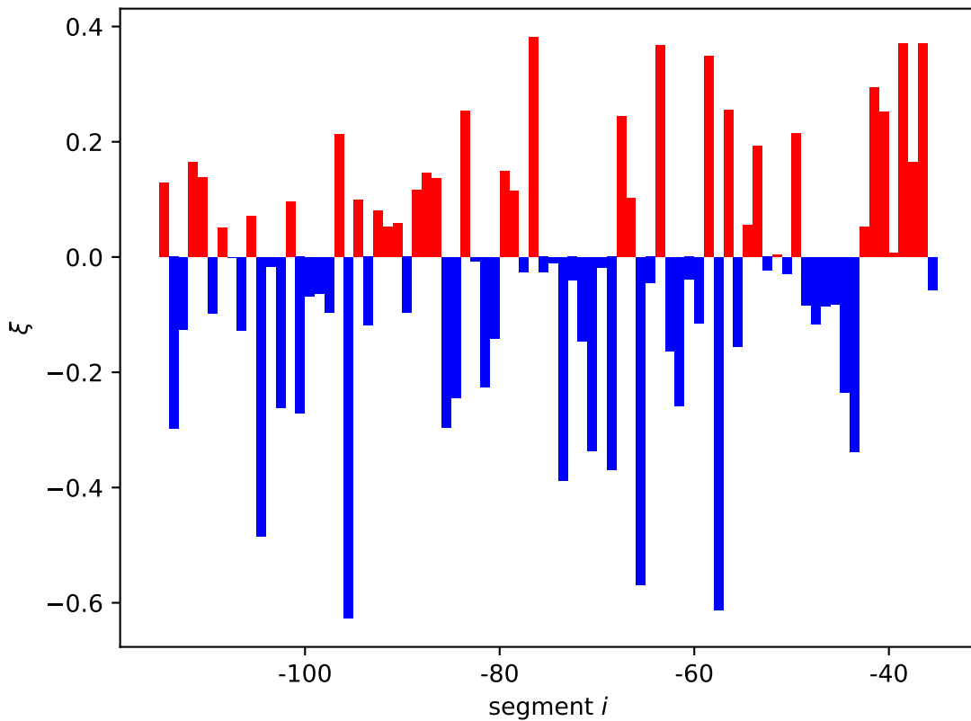
mscL expression shift \xi_i[11]
