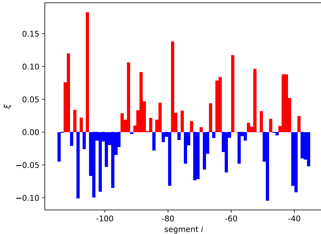
mscM expression shift \xi_i[11]
