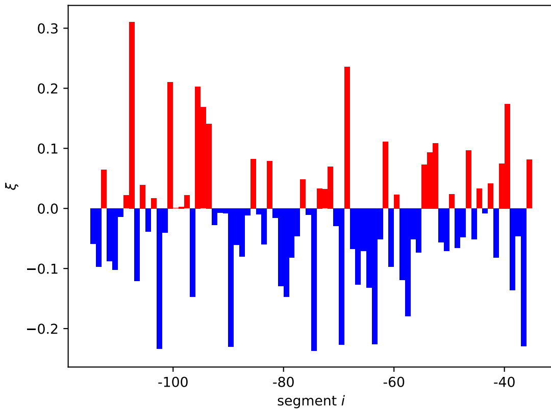
mscS expression shift \xi_i[11]
