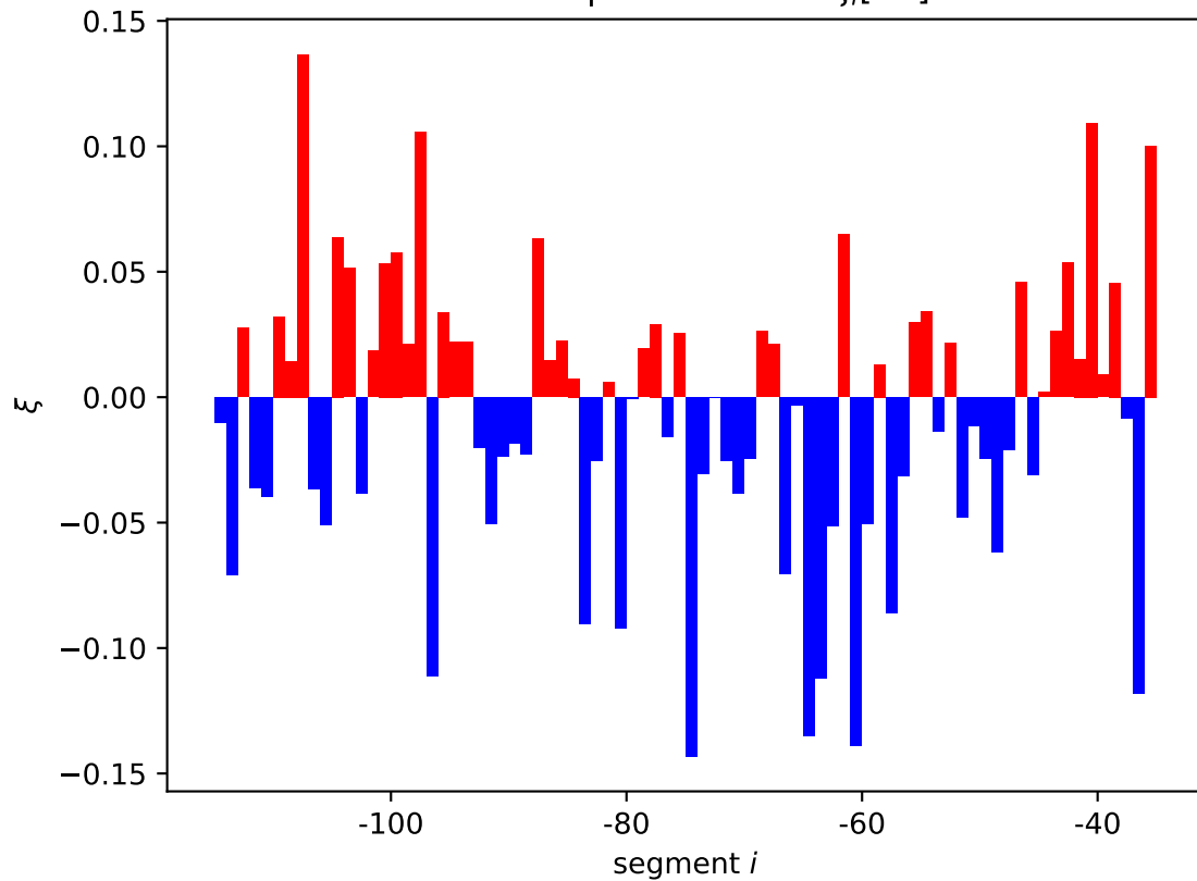
mscS expression shift \xi_i[11]
