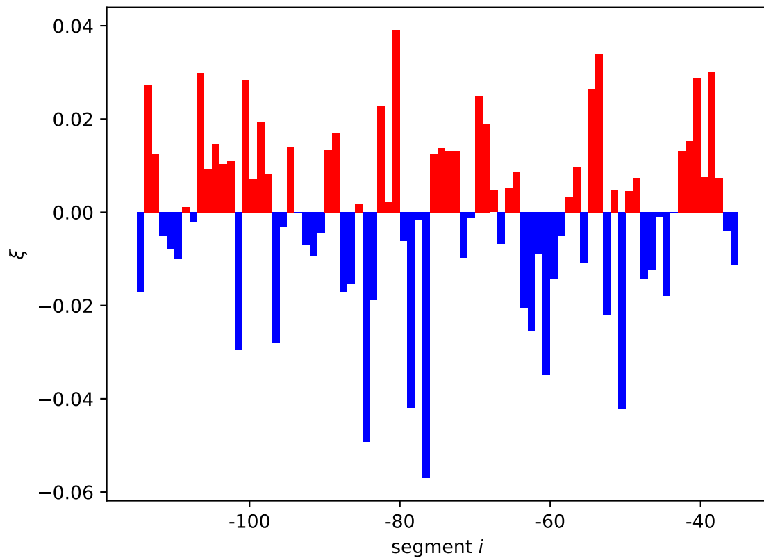
ompR expression shift \xi_i[01, 10]
