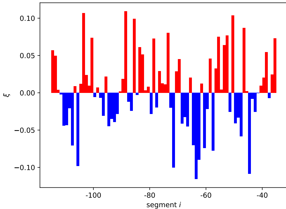
ompR expression shift \xi_i[11]
