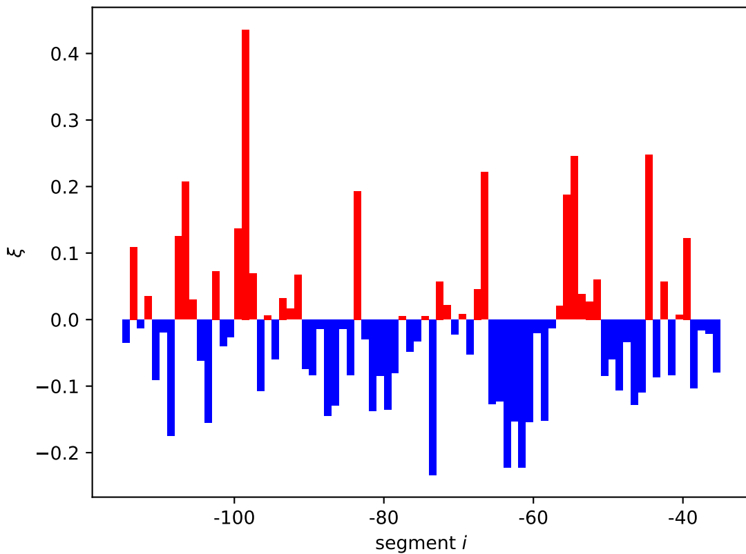
poxB expression shift \xi_i[11]
