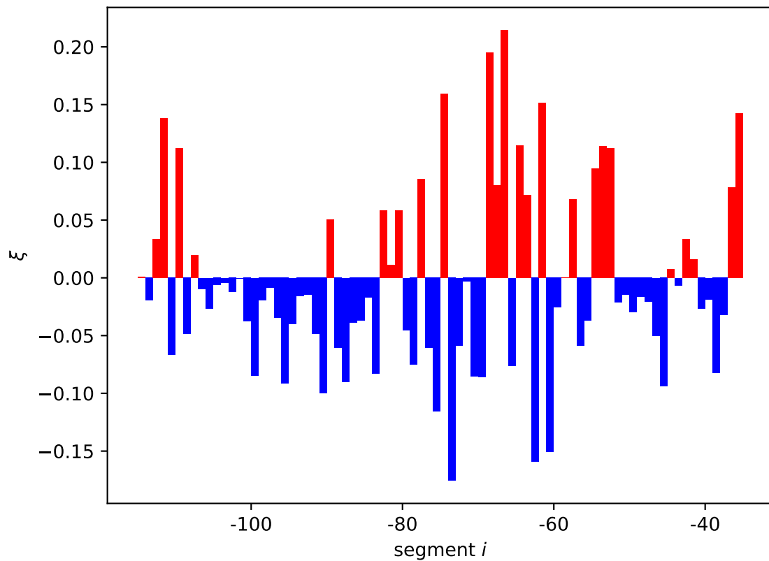
rapA expression shift \xi_i[11]
