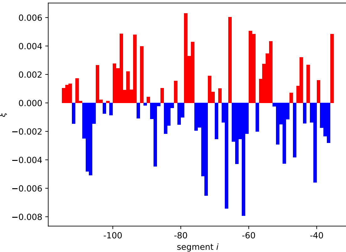
rumB expression shift \xi_i[01, 10]
