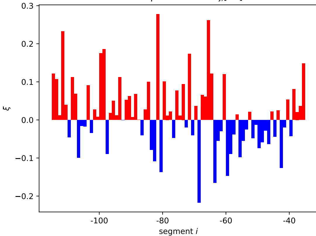
sbcB expression shift \xi_i[11]
