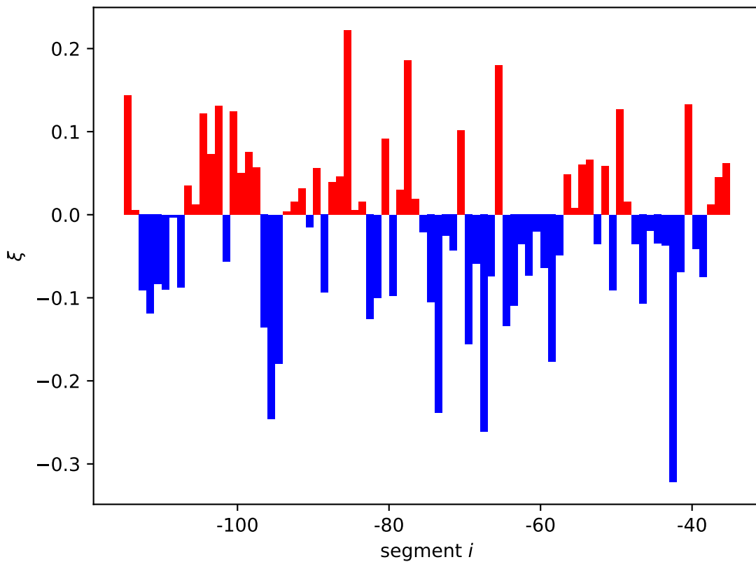
sdiA expression shift \xi_i[11]
