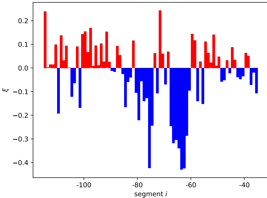
tff-rpsB-tsF expression shift \xi_i[11]
