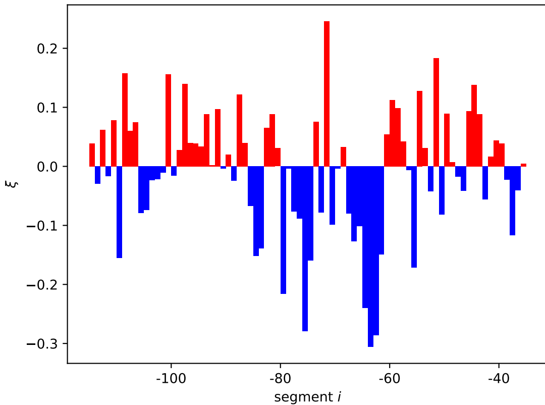
tff-rpsB-tsfc expression shift \xi_i[11]
