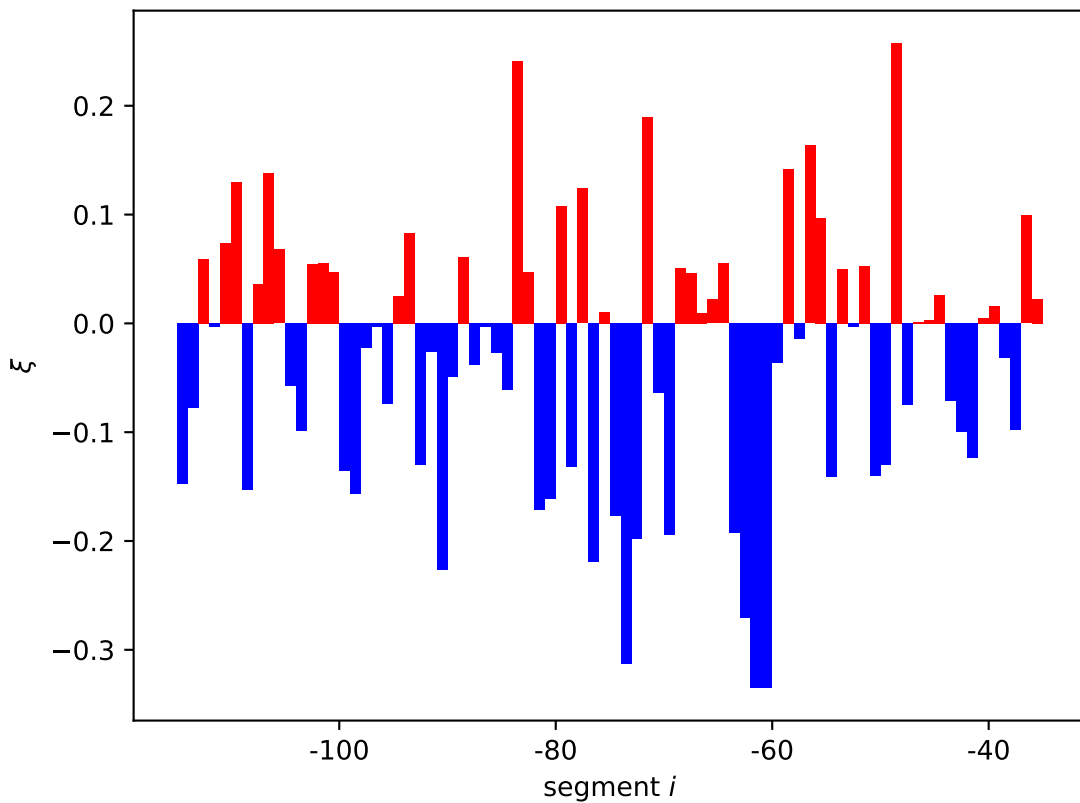
tig expression shift \xi_i[11]
