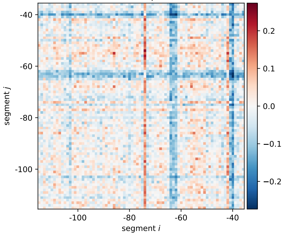
uvrD expression shift \xi_{i,j}[0101, 0110, 1010]
