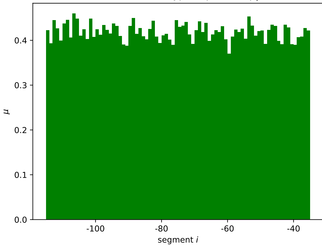
uvrD mean wildtype expression \mu_i^*
