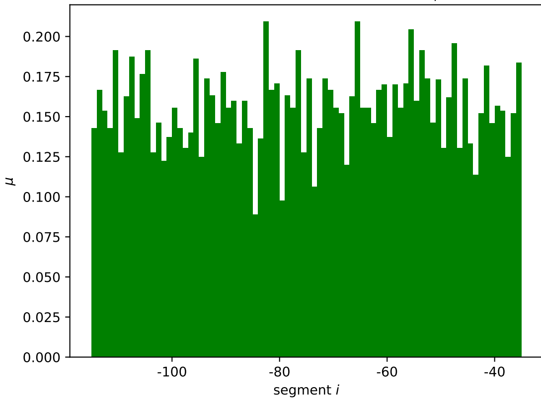
uvrD mean wildtype expression \mu_i^*
