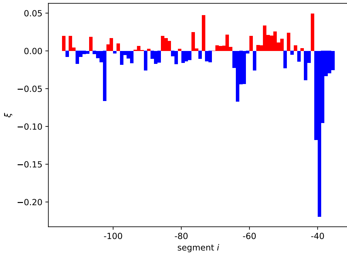
uvrD expression shift \xi_i[01, 10]
