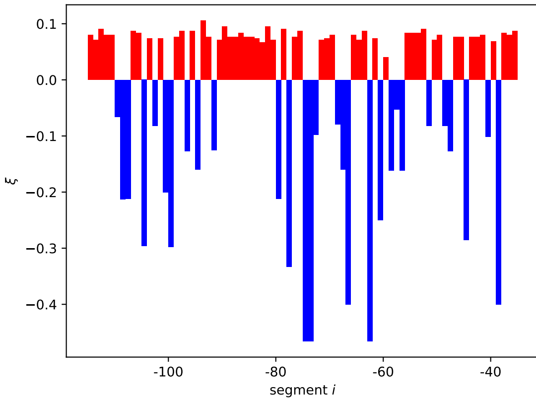
xapAB expression shift \xi_i[01, 10]
