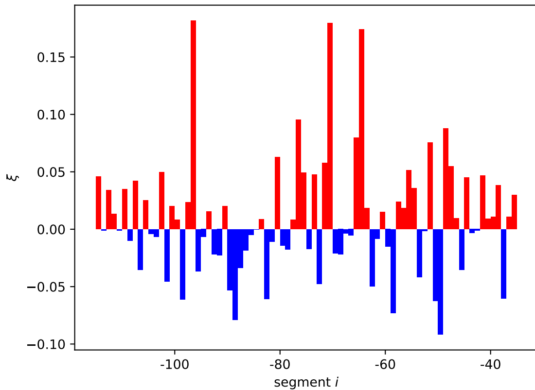
xapAB expression shift \xi_i[11]
