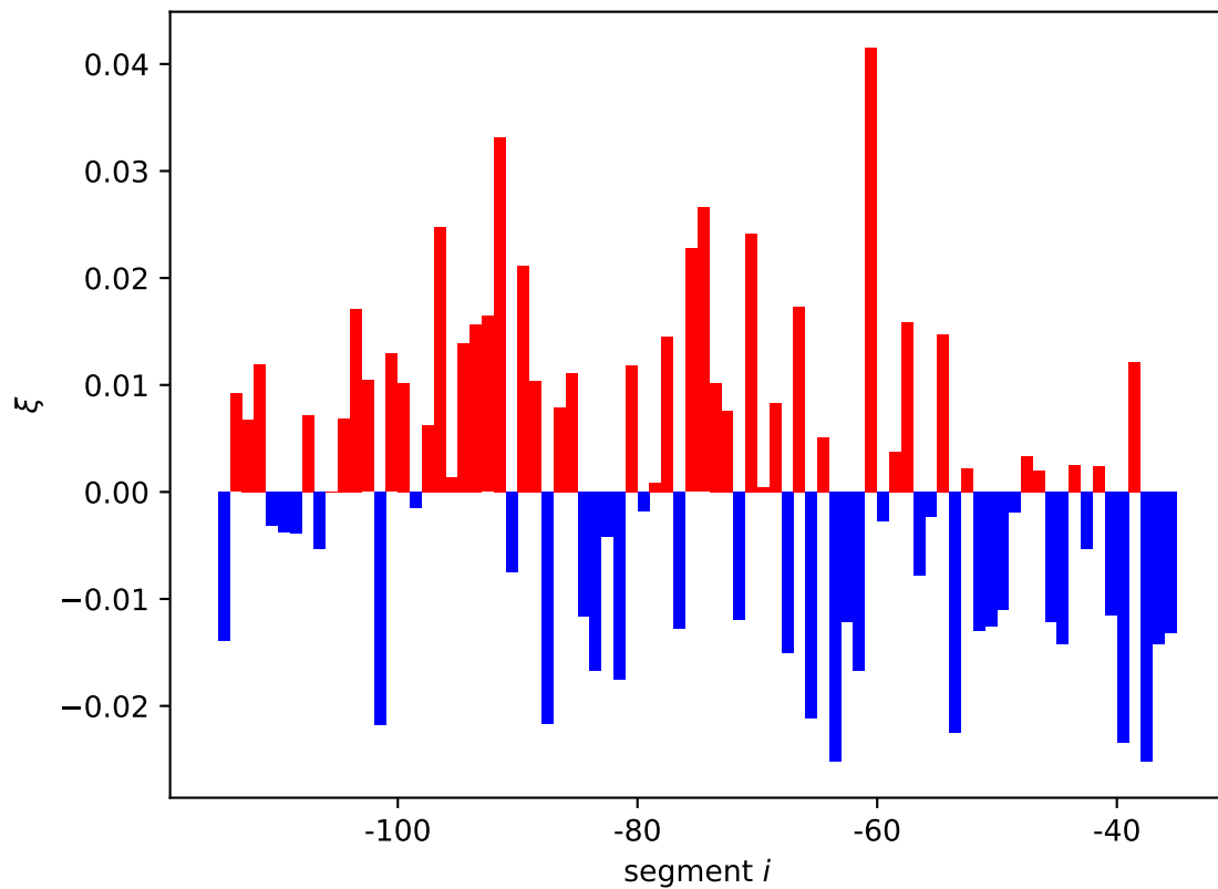
xapAB expression shift \xi_i[01, 10]
